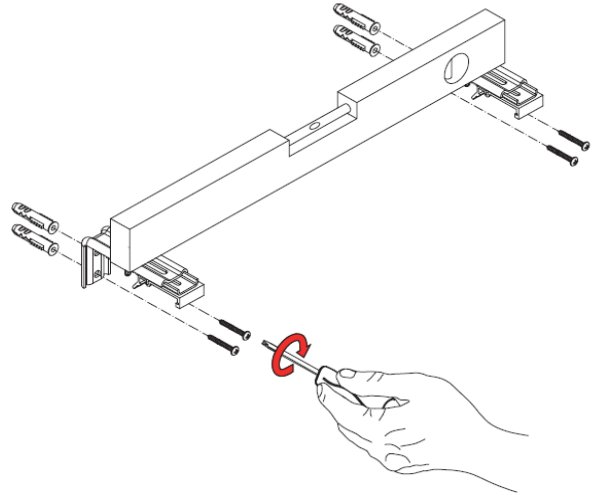
2 Waterpas stellen van de beugels
