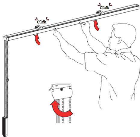
5 plaatsen van de rails
